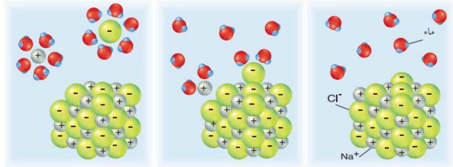
الشكل ٧ الماء يذيب ملح الطعام؛ لأن شحناته الجزيئية تنجذب نحو الأيونات المشحونة في الملح.
