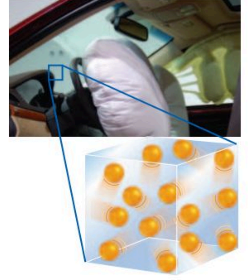
الشكل ٦ تتحرك جسيمات الغاز في جميع الاتجاهات بسرعة عالية. وينتشر الغاز بسرعة ليملأ حيز الوسادة.
