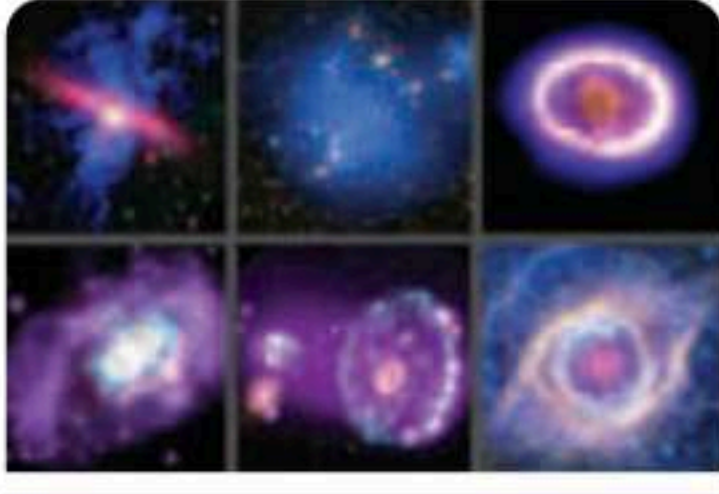
الشكل 17-3 صور لسدم بنطاق الأشعة السينية بواسطة مرصد شاندرا. المصدر: وكالة ناسا.
