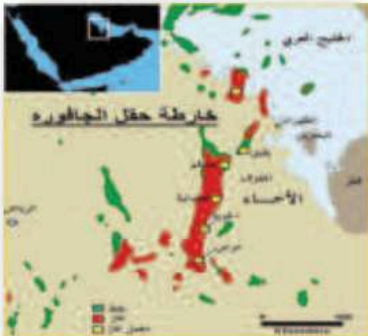
خارطة حقل الجافورة الجيولوجية.
