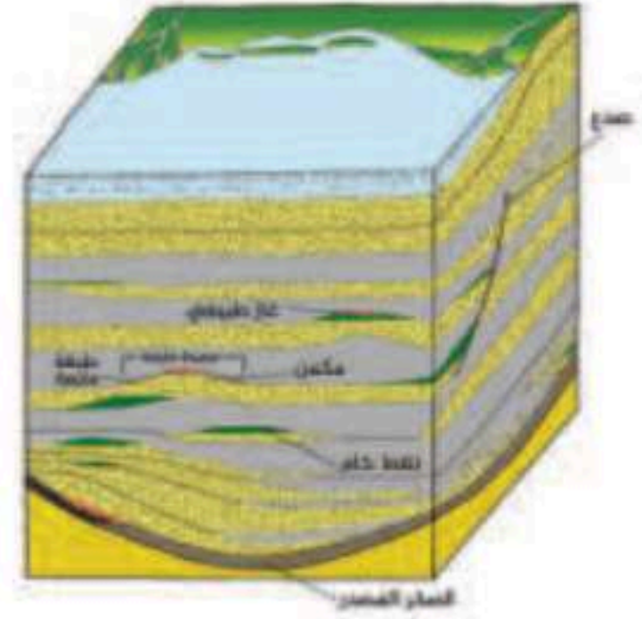
الشكل 2-5 صخر المصدر.
