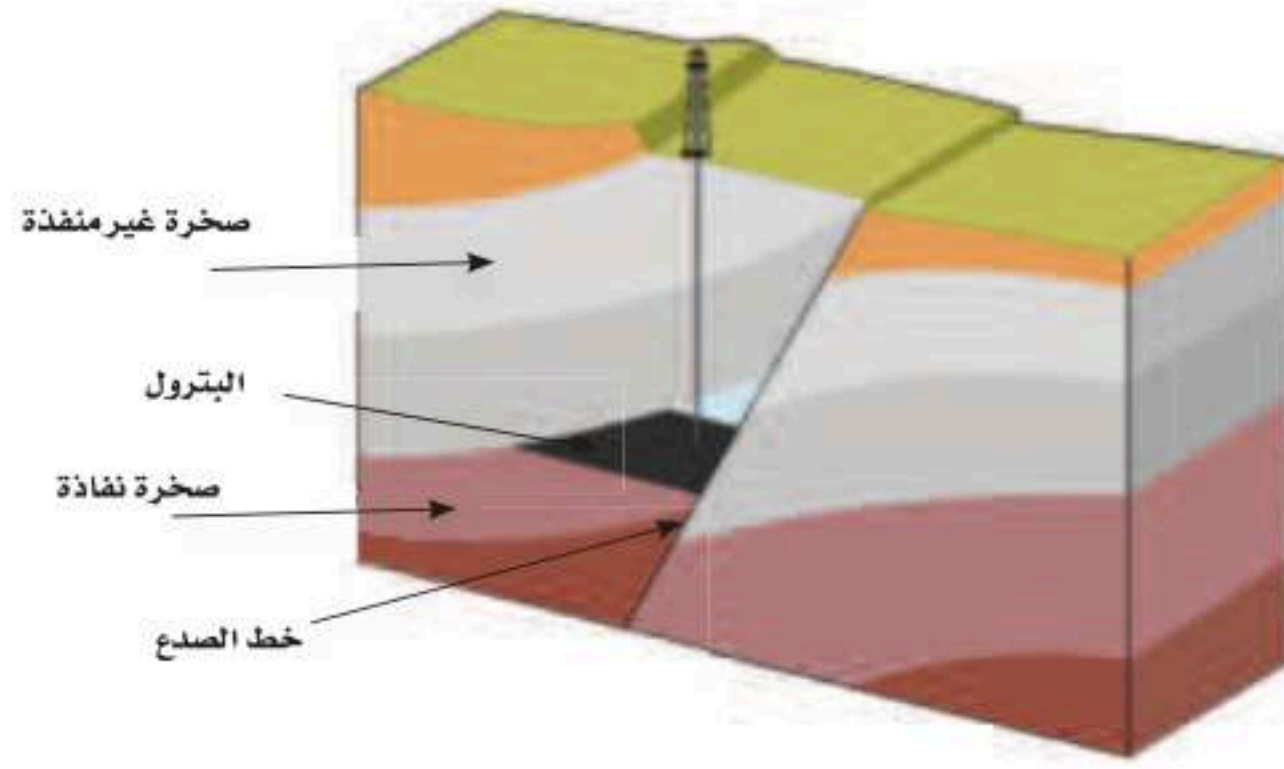
الشكل 4-5 مصائد الصدوع.
