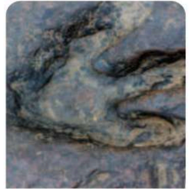
الشكل 4-8 آثار طبع أقدام الديناصورات.
