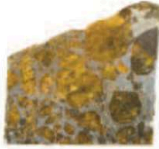
الشكل 17-1 نيزك صخري - حديدي.
