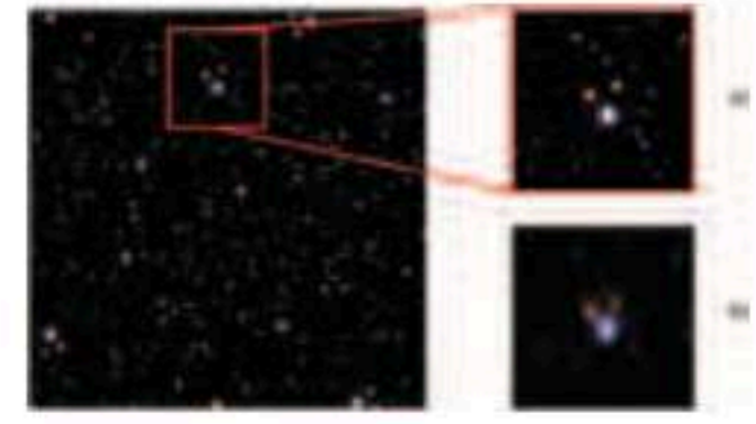
الشكل 10-3 صورة توضح الزيف الهالي.
