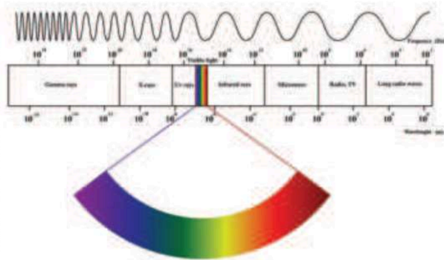
الشكل 1-3 نطاقات الطيف الكهرمغناطيسي.
