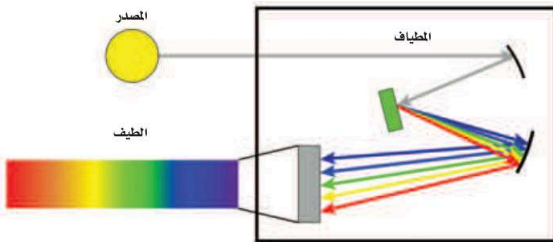
الشكل 2-3 تحليل الضوء بالمطياف.
