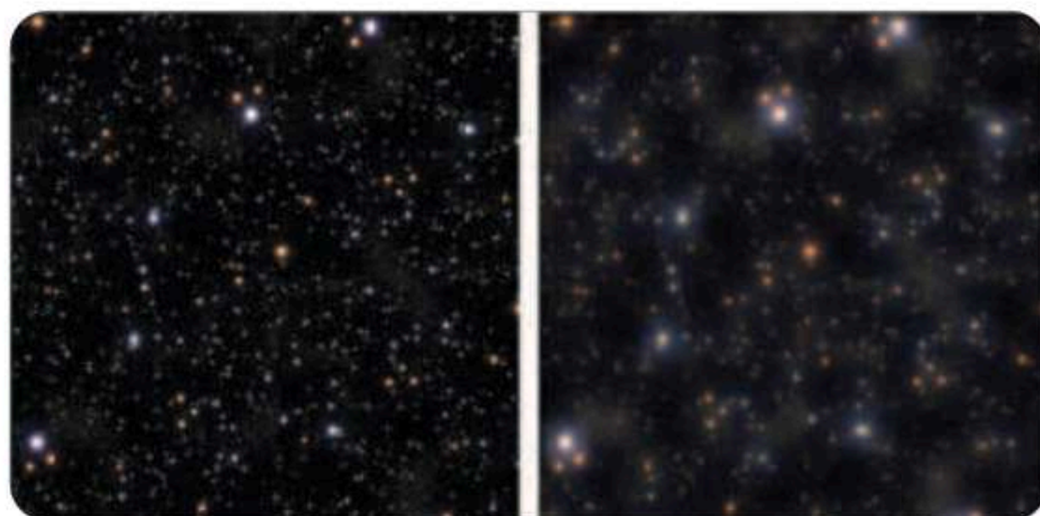
الشكل 3-8 صورة توضح الزيغ الكروي.
