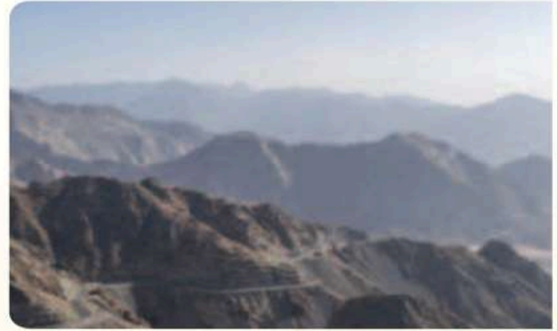
تشكلت سلسلة جبال السروات التي تمتد غرب الجزيرة العربية بفعل سلسلة من الأحداث المشكلة للأرض.
