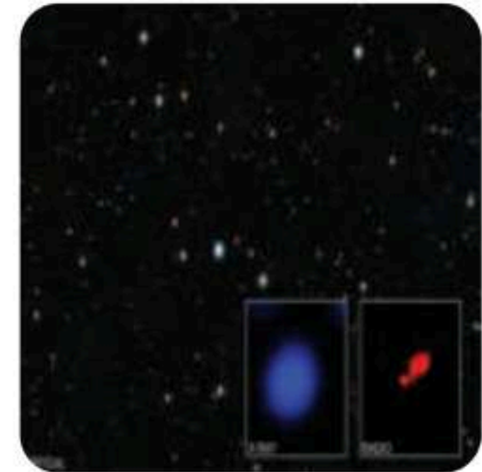
الشكل 16-3 كوازارات. المصدر: وكالة ناسا.
