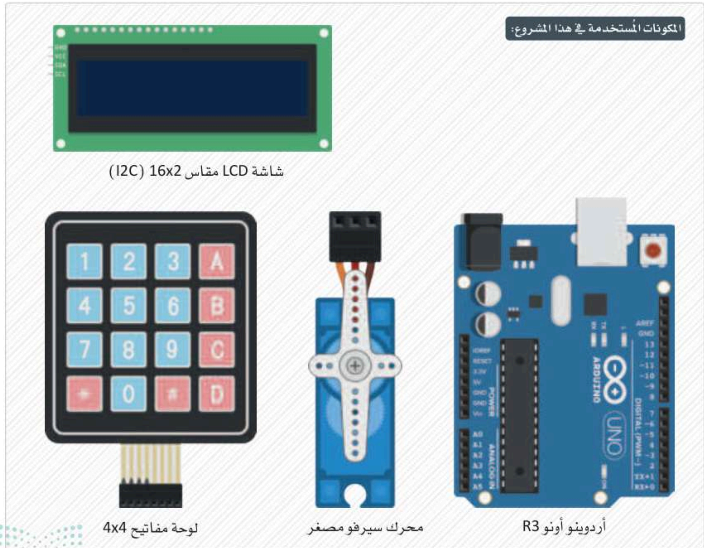
شكل 6.17: مكونات المشروع
