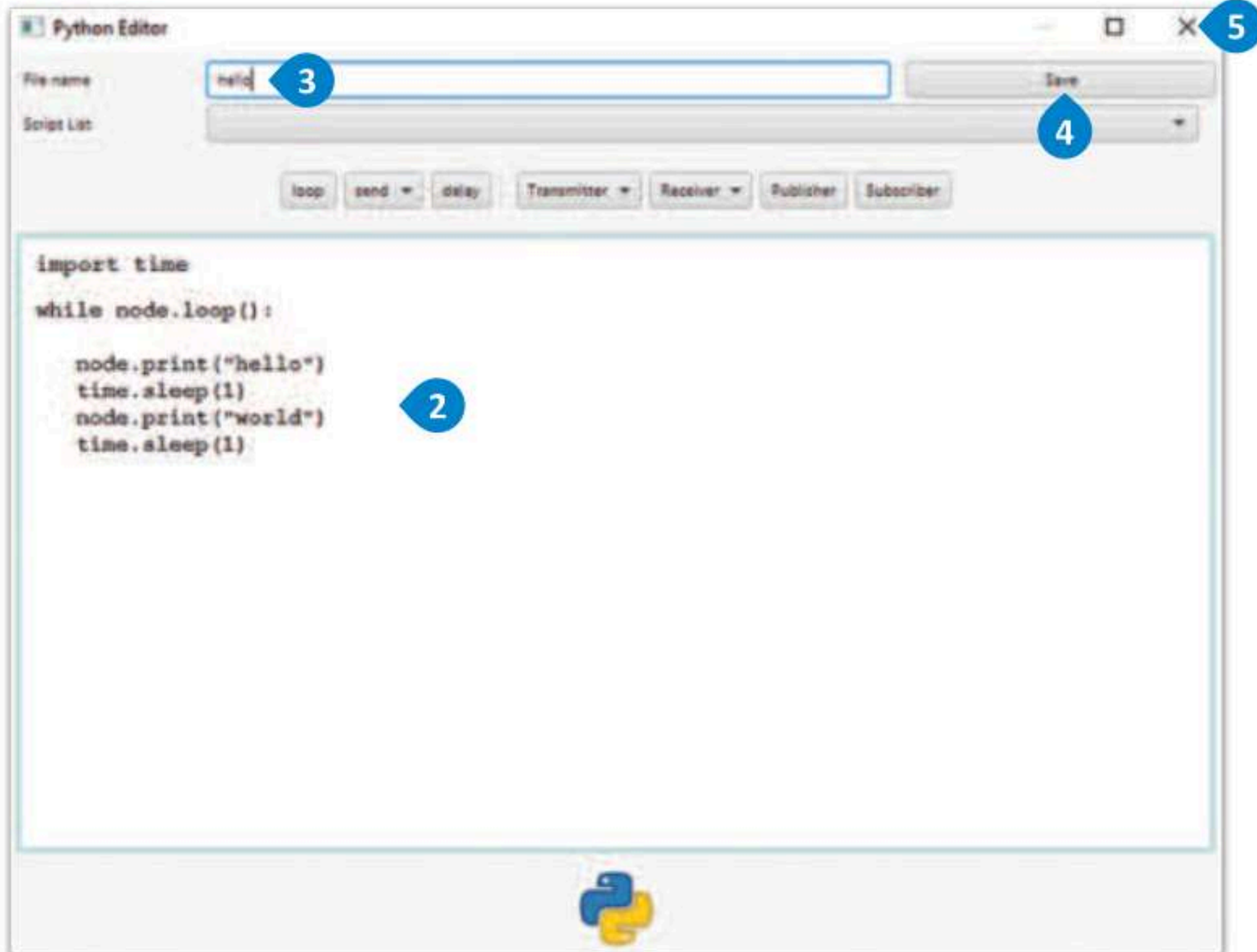
شكل 8.9: مُحرر البايثون
