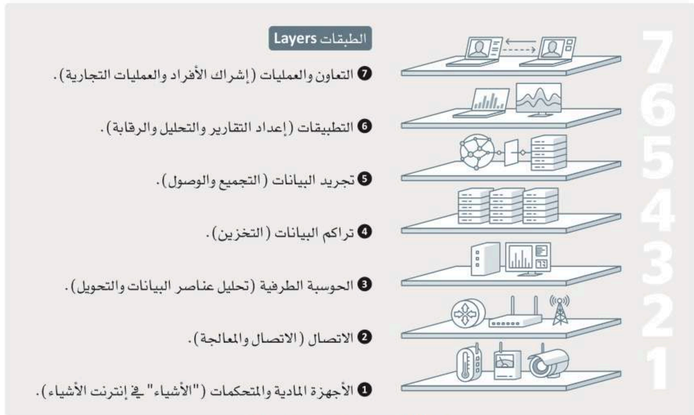
شكل 5.14: طبقات هيكلية إنترنت الأشياء العالمي
