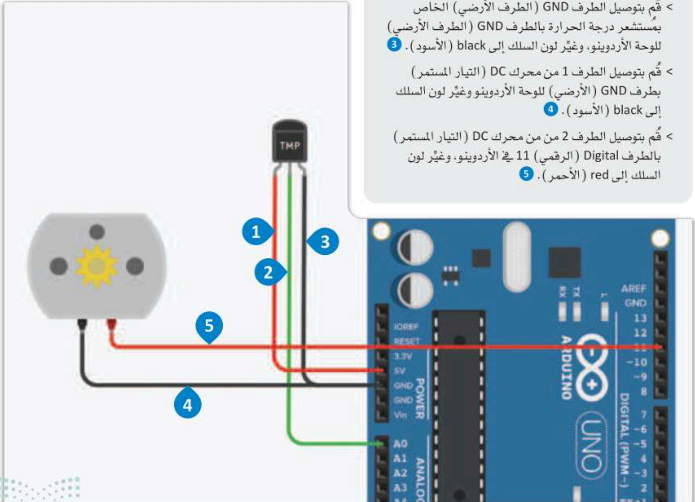
شكل 6.16: توصيل الدائرة
