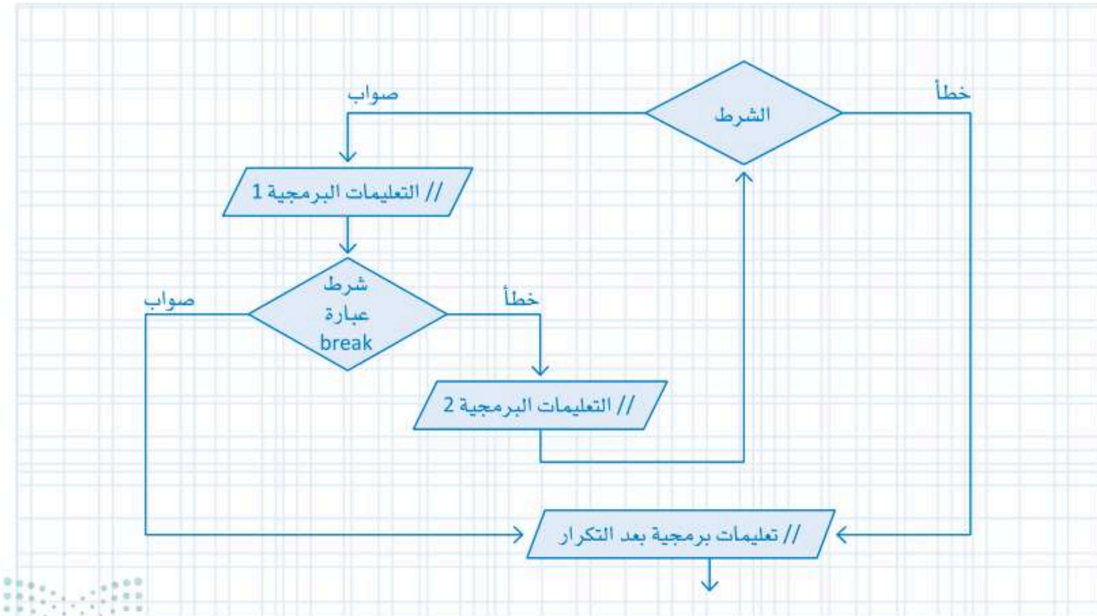
شكل 6.8: مخطط عبارة break
