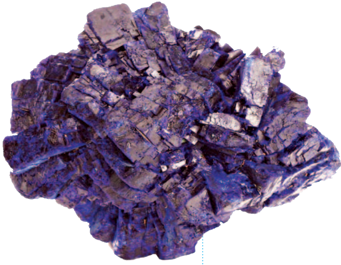
الشكل ٢ هذا التجمع من بلورات معدن الفلوريت تكوّن من محلول مشبع بمعادن ذائبة فيه.
