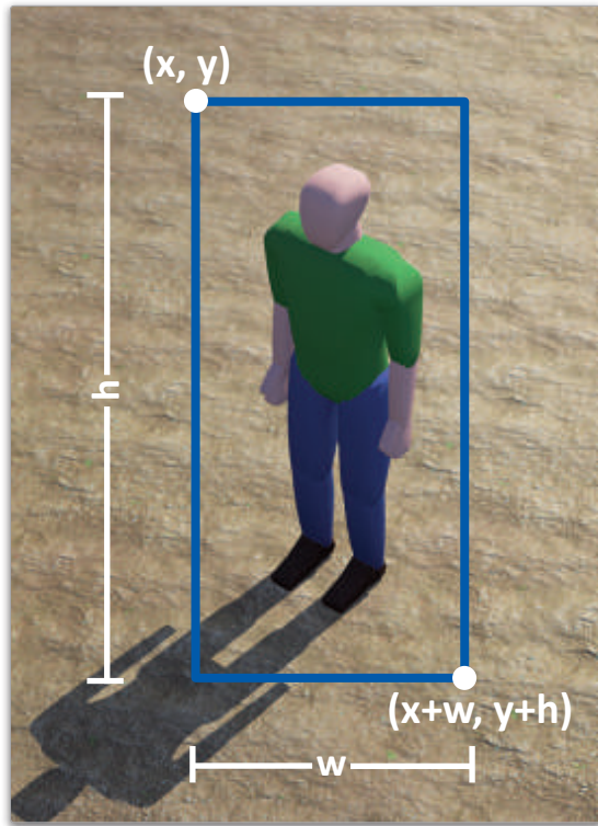
شكل 6.20: مُتغيّرات المستطيل
