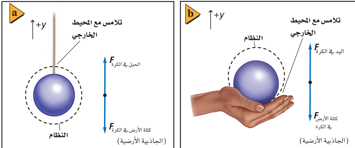
■ الشكل 4-2 2-4 لعمل نموذج فيزيائي للقوى المؤثرة في جسم، استخدم مخطط الجسم الحر، وارسم سهمًا لتمثيل كل قوة من القوى المؤثرة في الجسم، ثم سمّ القوة ومسببها.
