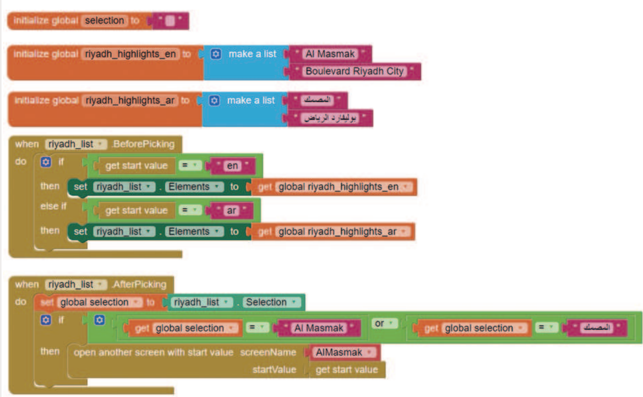
شكل 3.41: البرنامج بأكمله للشاشة الثانية
