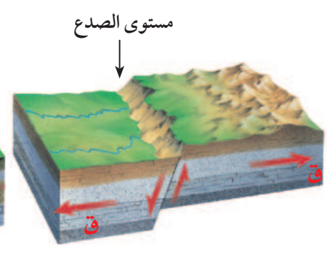
ج ينتج الصدع الجانبي (الإنزلاقي) عندما تتعرض الصخور لإجهادات قص (تؤثر فيها بصورة جانبية).
