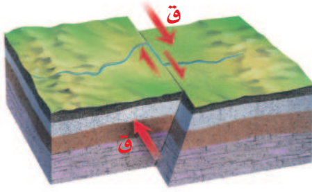
أ ينتج الصدع العادي عندما تسحب الصخور من الجانبين تحت تأثير إجهادات الشد (قوى الشد).
