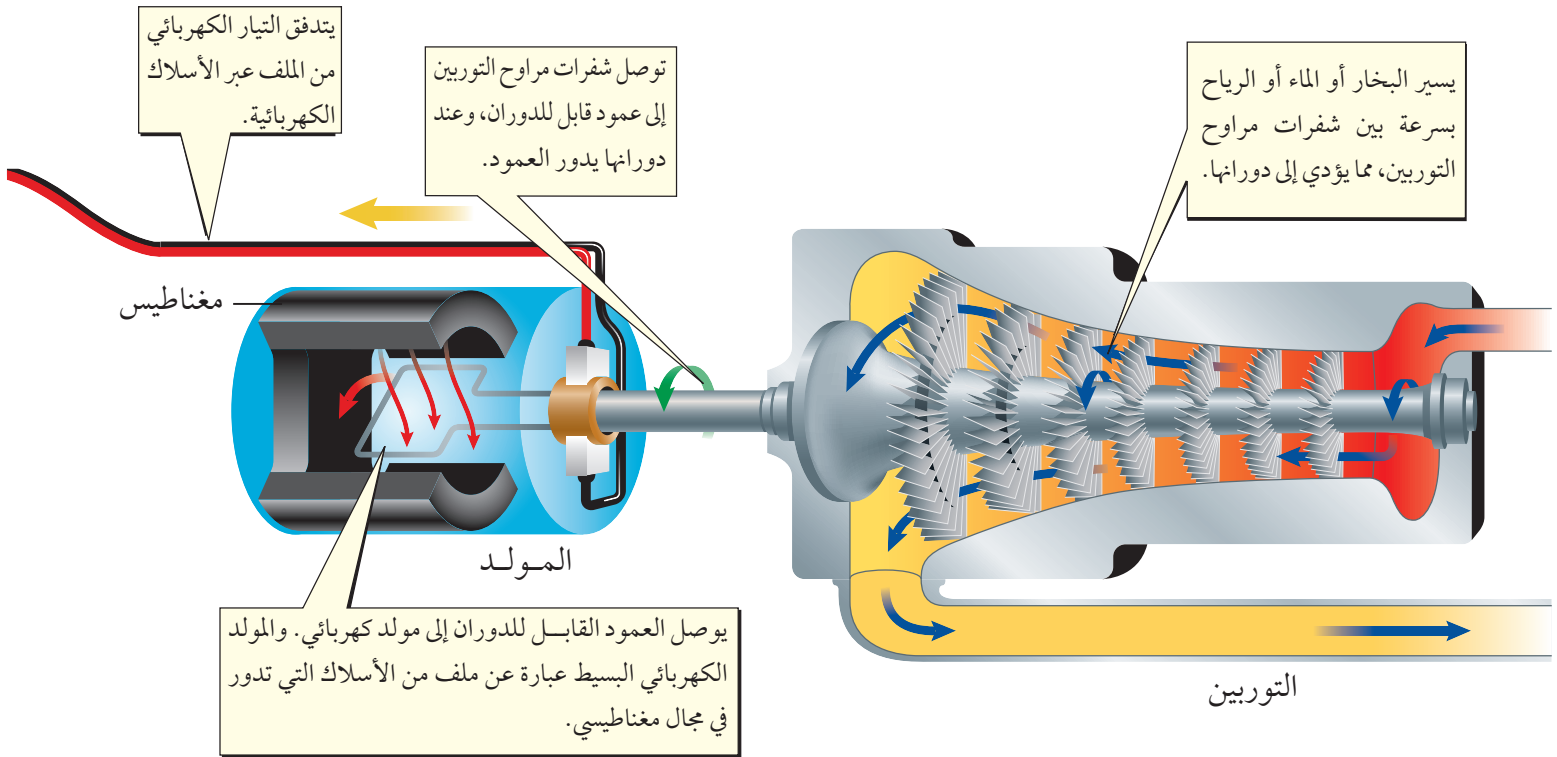
الشكل ١٤ تستخدم محطات توليد الطاقة المولدات لإنتاج الطاقة الكهربائية، وفي محطات الوقود الأحفوري يحرق الوقود الأحفوري ليعمل على غلي الماء لإنتاج البخار الذي يحرك تروس التوربينات.
