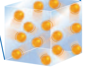
الشكل ٦ تتحرك جسيمات الغاز في جميع الاتجاهات بسرعة عالية. ويتنشر الغاز بسرعة ليملاً حَيَرِ الوسادة.
