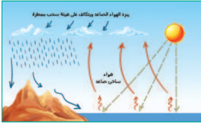
المطر التصاعدي
