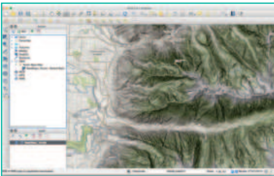
برنامج QGIS
