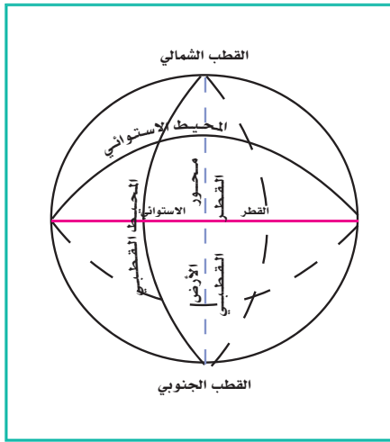
أبعاد الأرض
