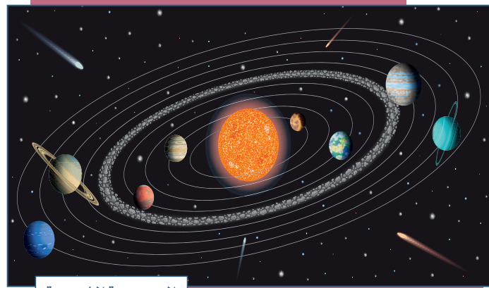
المجموعة الشمسية
